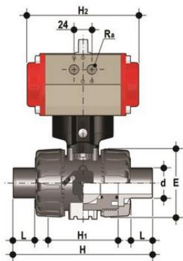
Шаровой кран VKD с пневмоприводом ДвД с втулочными окончаниями (уплотнение FKM) PP-H d50 (DN40)
