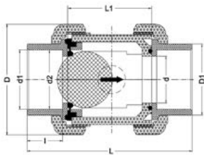
Обратный клапан шаровой с муфтовыми окончаниями PP-H IPS (FKM) d75
