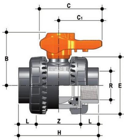
Шаровой кран общего применения VXE ХПВХ с резьбовыми окончаниями R2" (DN50)
