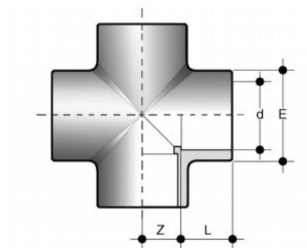
Крестовина клеевая ПВХ FIP d40
