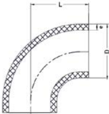
Отвод для стыковой сварки 90° PP-H IPS d315 PN10
