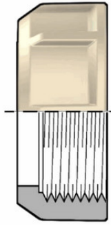
Гайка ПВДФ 1 1/4 SDR21 PN16
