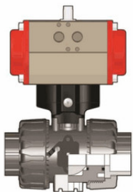
Шаровой кран VKD ПВХ с пневмоприводом НЗ с муфтовыми окончаниями, EPDM, FIP d16 (DN10)
