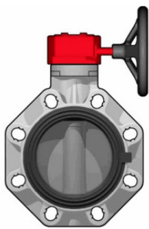
Дисковый затвор ПВХ FKOAVRM с редуктором, EPDM, FIP d16" (DN400)
