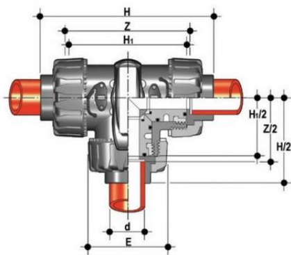
3-х ходовой шаровой кран ТКД с муфтовыми окончаниями L-шар (уплотнение EPDM) PP-H d63 (DN50)
