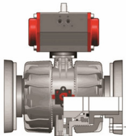
Шаровой кран VKD с пневмоприводом ДвД с фланцевыми окончаниями, DN65-100 (уплотнение EPDM) PP-H d75 (DN65)
