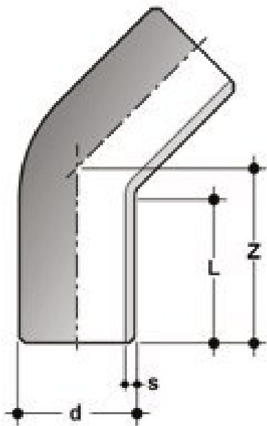
Отвод 45° для стыковой сварки PP-H FIP d225 SDR11 PN6
