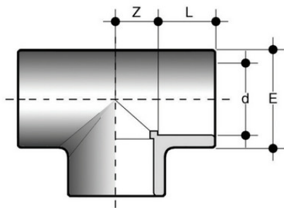
Тройник равнопроходной клеевой 90° ПВХ FIP d180
