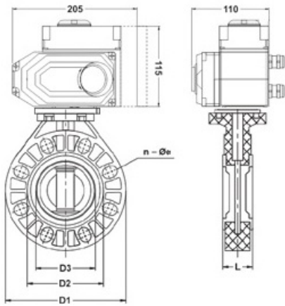
Дисковый затвор IFK ПВДФ с электрическим приводом 220V AC, FKM, IPS d110 (DN100)
