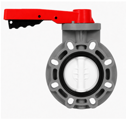
Затвор дисковый в корпусе FRPP (диск - ПВДФ) с рукояткой промышленного применения FKM IPS d160 (DN150)
