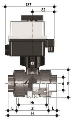
Шаровой кран для регулирования потока VKR ПВХ с эл.приводом 24V AC 12VDC, муфтовые окончания, EPDM, FIP d32 (DN25)
