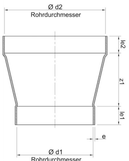
Муфта переходная PPs 630x450
