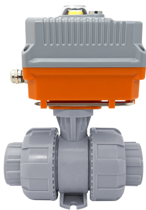
Шаровой кран IVKD ХПВХ с эл.приводом 220V AC, муфтовые окончания d90 (DN80)
