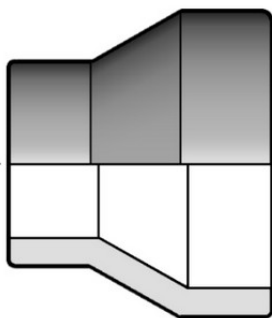
Муфта редукционная для стыковой сварки PP-H FIP (PN10) 63x32 SDR11 PN10
