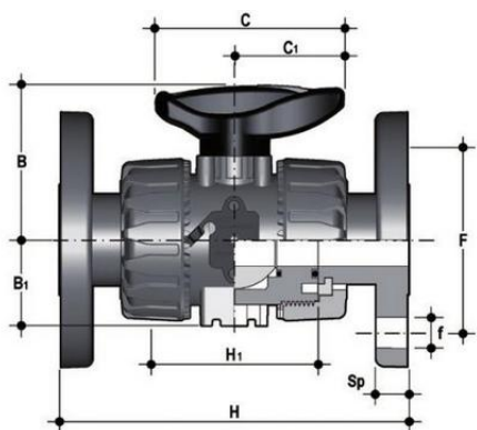
Шаровой кран промышленного применения VKD с фланцевыми окочаниями (уплотнение EPDM) PP-H d50
