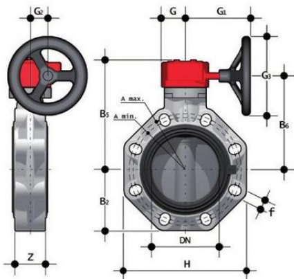
Дисковый затвор FK ХПВХ с редуктором d110 (DN90)
