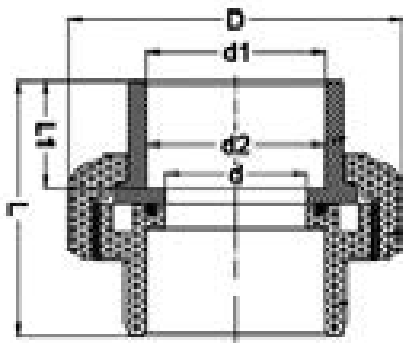
Муфта ХПВХ IPS (Model B) d15 PN16
