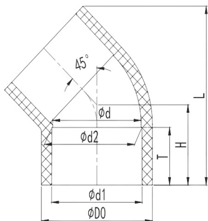
Отвод клеевой 45° ПВХ IPS d355
