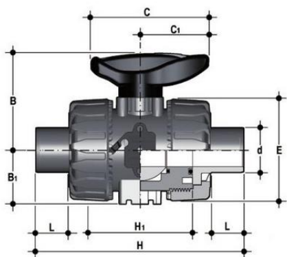
Шаровой кран промышленного применения VKD со втулочными окончаниями (уплотнение FKM) PP-H d50 (DN40)
