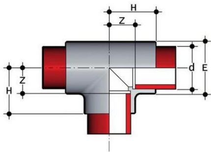
Тройник равнопроходной для раструбной сварки PP-H FIP d75 PN10
