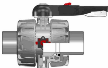
Шаровой кран VKD ПВДФ с втулочными окончаниями, DN65-100 d75 (DN65)
