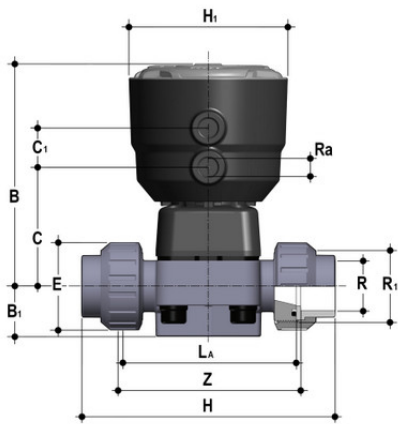
Мембранный клапан ДК ПВХ с пневмоприводом НЗ, PN6, муфтовые окончания, EPDM, FIP d25 (DN20)
