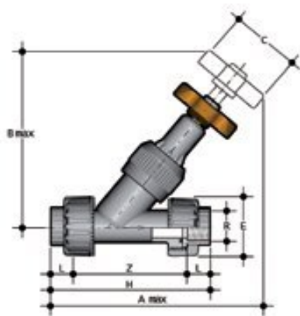
Угловой вентиль VVUFV PBX с резьбовыми окончаниями, EPDM, FIP R3/4" (DN20)
