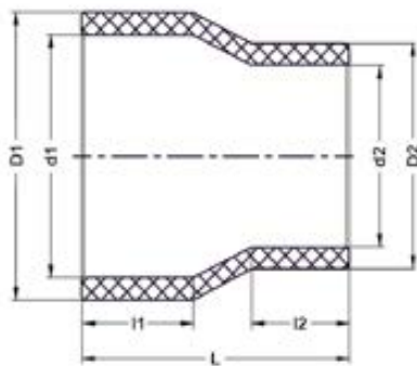
Муфта переходная для стыковой сварки РР-Н IPS (Model A) 32x25 PN10
