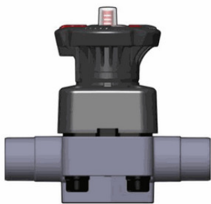
Мембранный клапан DK с втулочными окончаниями (уплотнение FKM / мембрана FKM) PP-H d20 (DN15)
