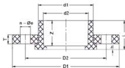
Фланец свободный с буртом ХПВХ IPS (Model B) - комплект d280 PN10
