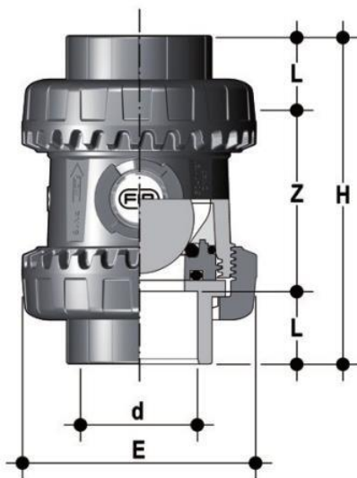
Шаровой обратный клапан SXEIV ПВХ; с муфтовыми окончаниям, FKM, FIP d32 (DN25)
