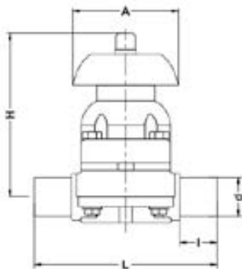
Мембранный клапан IDK ПБХ с втулочными окончаниями, EPDM, IPS d40 (DN32)
