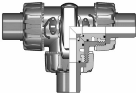
3-х ходовой шаровой кран ПВХ ТКД с втулочными окончаниями, L-шар, FKM, FIP d20 (DN15)
