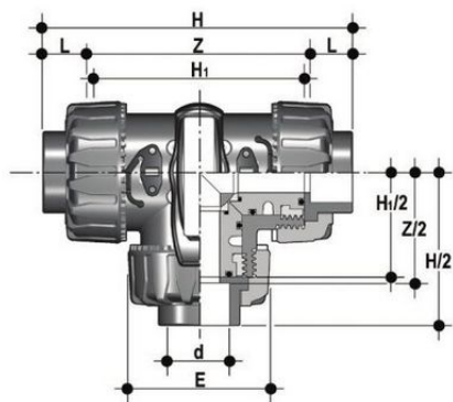
3-х ходовой шаровой кран ПВХ ТКД с муфтовыми окончаниями, L-шар, FKM, FIP d32 (DN25)
