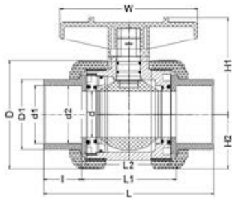
Кран шаровой промышленного применения с муфтовыми окончаниями PP-H IPS d32
