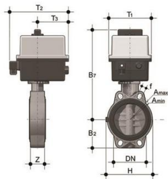
Дисковый затвор общего применения FE ПВХ с эл.приводом 24V AC/DC, EPDM, FIP d110 (DN100)
