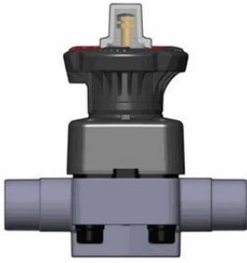
Мембранный клапан DKLDV ПВХ с муфтовыми окончаниями, EPDM, FIP d63 (DN50)
