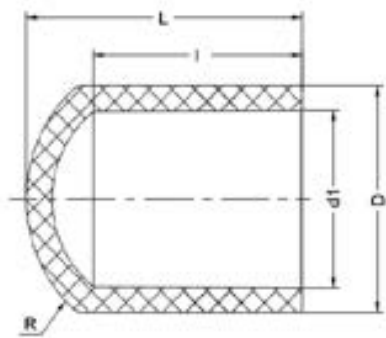
Заглушка ПВДФ для стыковой сварки d50 PN 16
