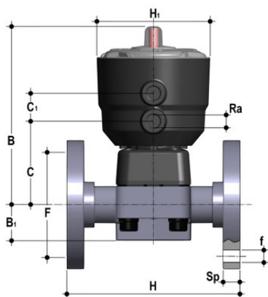
Мембранный клапан ДК ПВДФ с пневмоприводом ДвД, PN10 с фланцевыми окончаниями d50 (DN40)
