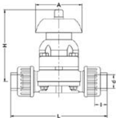
Мембранный клапан с муфтовыми окончаниями PP-H IPS d20 (DN15)
