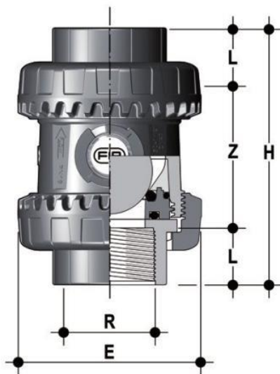
Шаровой обратный клапан SXEFV ПВХ; с резьбовыми окончаниям, FKM, FIP R1/2" (DN15)
