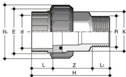
Муфта разборная переходная ХПВХ/ нержавеющая сталь НР 20х1/2" PN16
