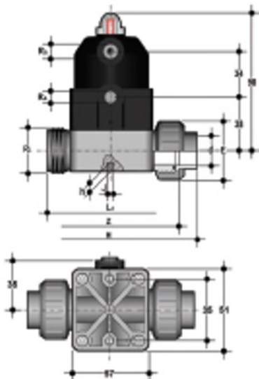
Компактный мембранный клапан ПВХ с пневмоприводом, CM, EPDM, FIP d20 (DN15)
