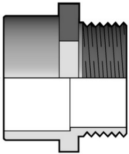
Адаптер с наружной резьбой PP-H FIP 32x1 SDR11 PN6
