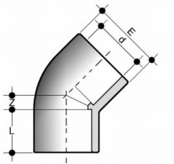
Отвод клеевой 45° ПВХ FIP d20
