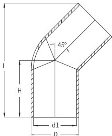
Отвод для стыковой сварки ПВДФ 45° d32 PN 16
