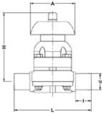
Мембранный клапан IDK ПВХ с втулочными окончаниями, EPDM, IPS d40 (DN32)
