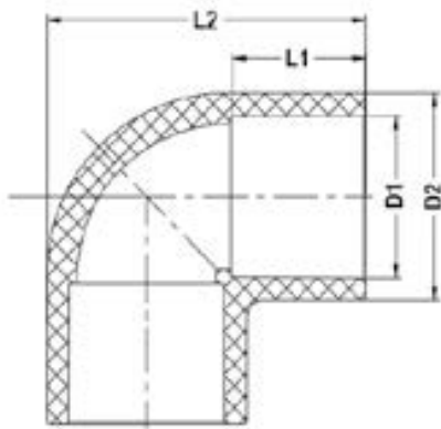
Отвод 90° ХПВХ IPS (Model A) d140 PN16
