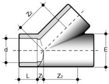
Тройник равнопроходной клеевой 45° PBX FIP d50
