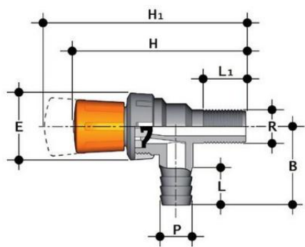
Мембранный кран RMRPV ПВХ, EPDM, FIP d15 (DN15)
